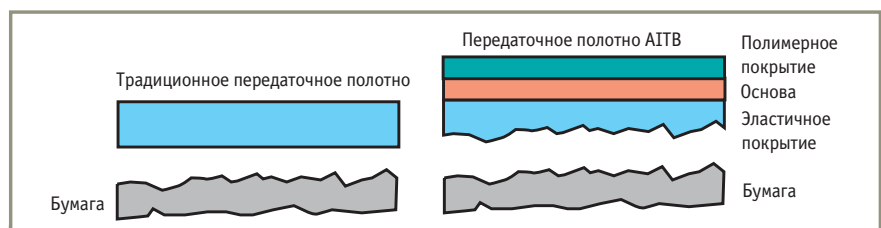
Рис. 7. Эластичная поверхность ленты переноса изображения (AITB) позволяет более точно повторять неровности бумаги и более равномерно наносить тонер
